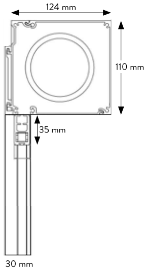
Acrimo 1302 110 x 120 mm kassette med bundskinne 18 x 35 mm
