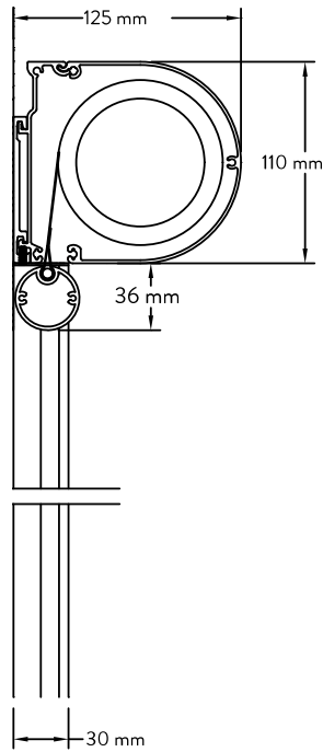
Acrimo 1900 D 110 mm kassette med rund bundskinne Ø 36 mm
