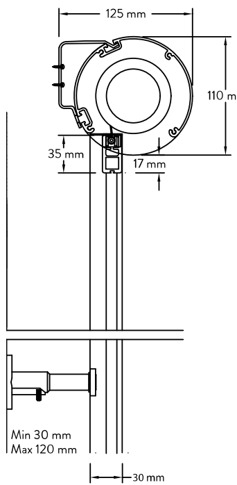
Acrimo 1400 Ø 110 mm kassette med bundskinne 18 x 35 mm
