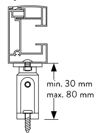
Væg montering med justerbar afstandsholder
