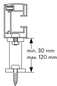
Væg montering med afstandsholder
